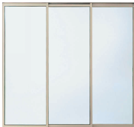
W9尺 3枚建 右勝手(W2,600×H2,430mm)
