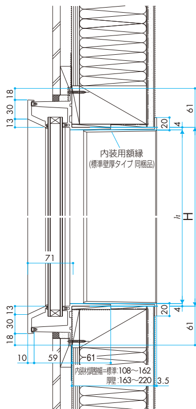
◎ A-A'断面
