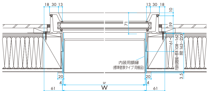
◎ B-B'断面
