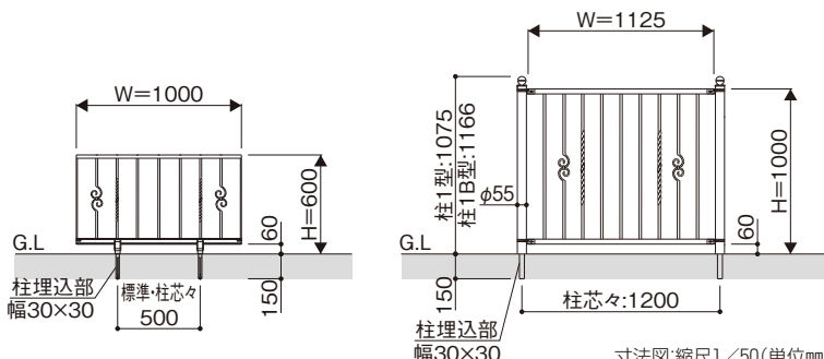
トラディションフィックスフェンス ▶P.892
