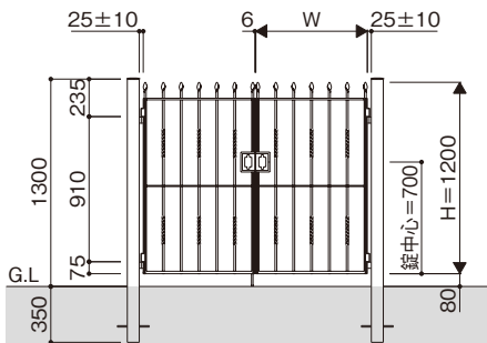
7B型: バスケットツイストタイプ
