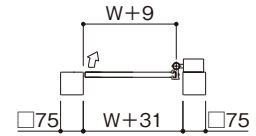
5B型:バスケットツイストタイプ
