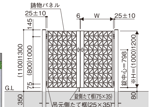
寸法図:縮尺1/50(単位:mm)
