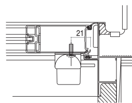
半外付型に取付時
